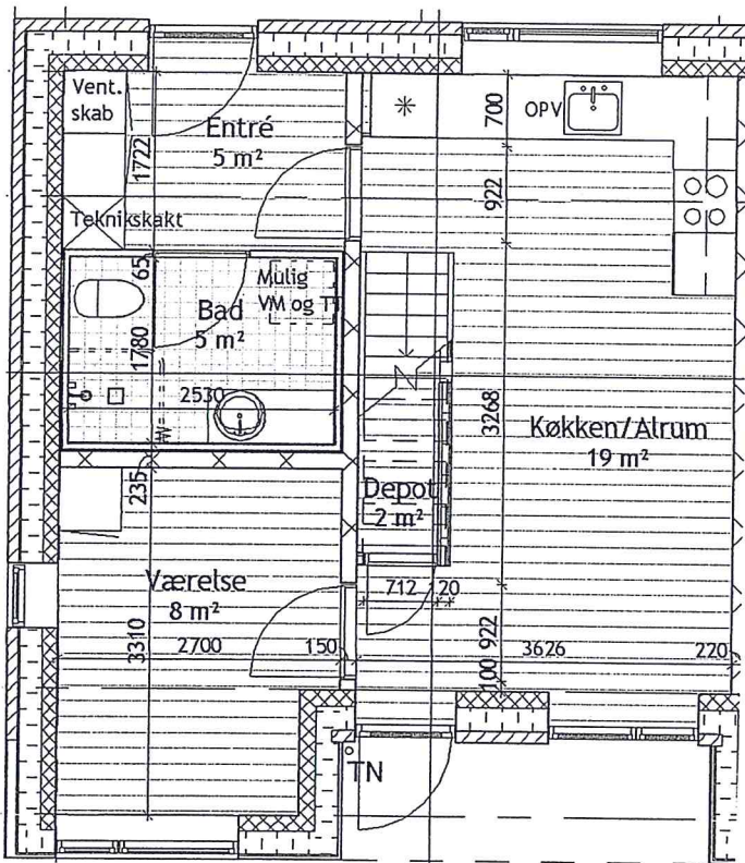
Stueetage
